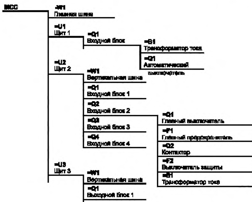
а) Древоидная структура, ориентированная на продукт
