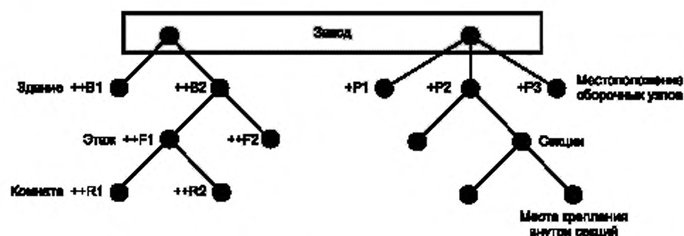
Рисунок F.4 — Структуры завода, ориентированные на местоположение
