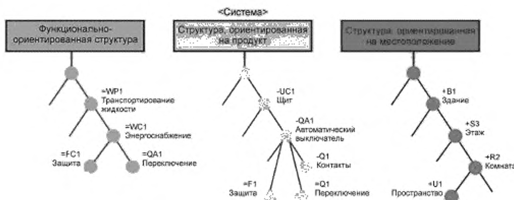
Рисунок С.9 — Структуры с обозначенными подобъектами
