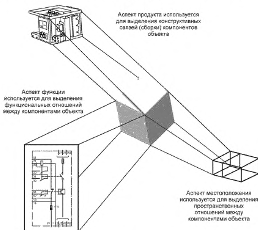
Рисунок 3 — Аспекты объекта
