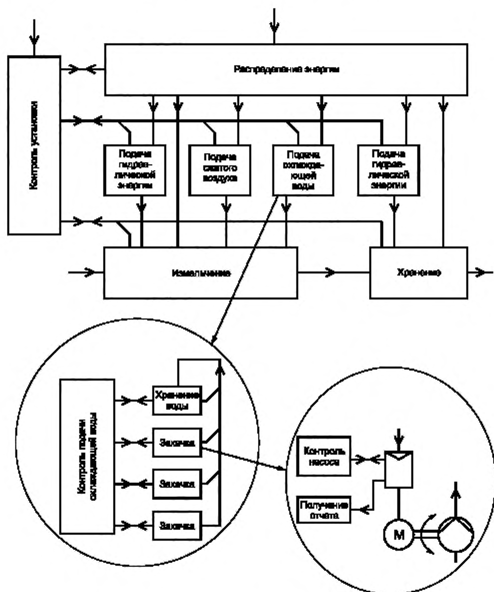
Рисунок 14 — Функционально-ориентированная структура
