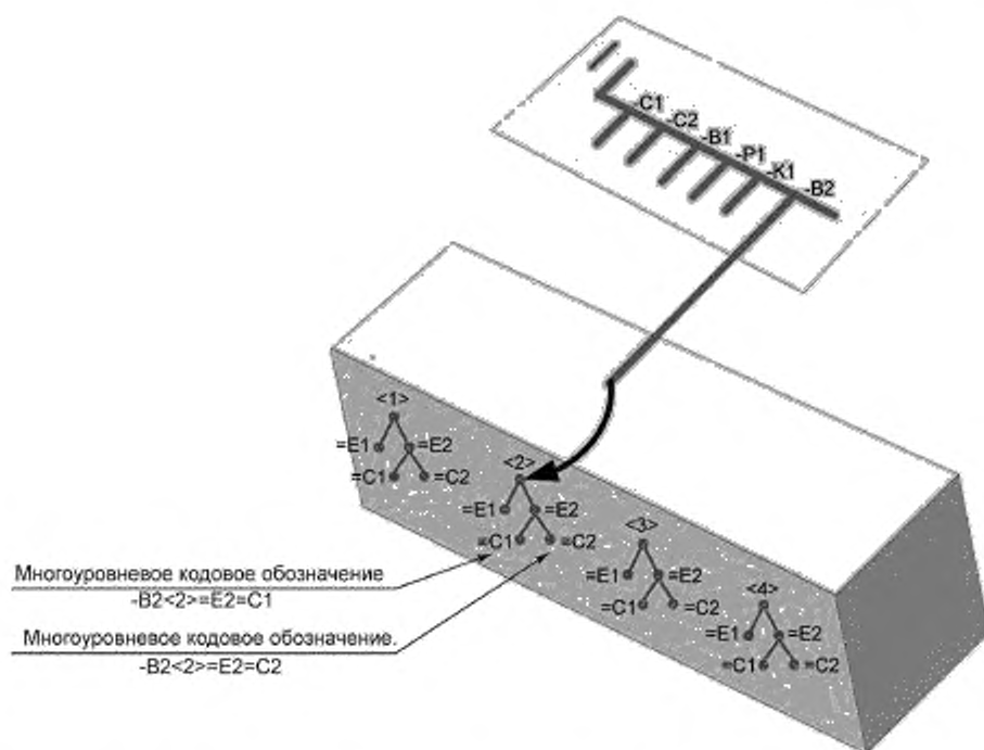
Рисунок Е.2 — Пример многоуровневых кодовых обозначений, использующих различные аспекты объекта с несколькими независимыми верхними узлами в одном аспекте
