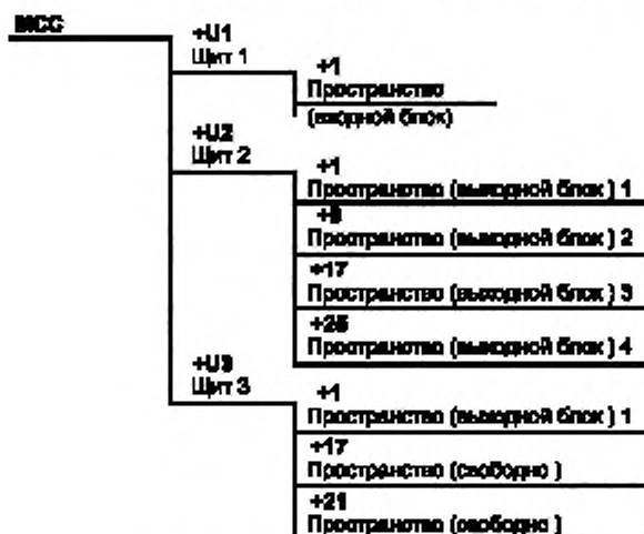
б) Древоидная структура, ориентированная на местоположение
