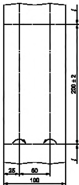
Рисунок В.1 — Складывание образца для испытаний
