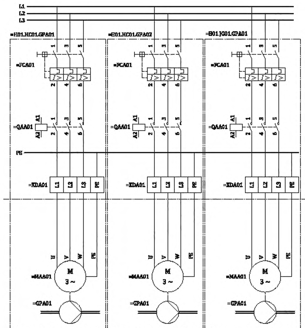
Рисунок В.23 — Схема электроснабжения трех насосных установок
