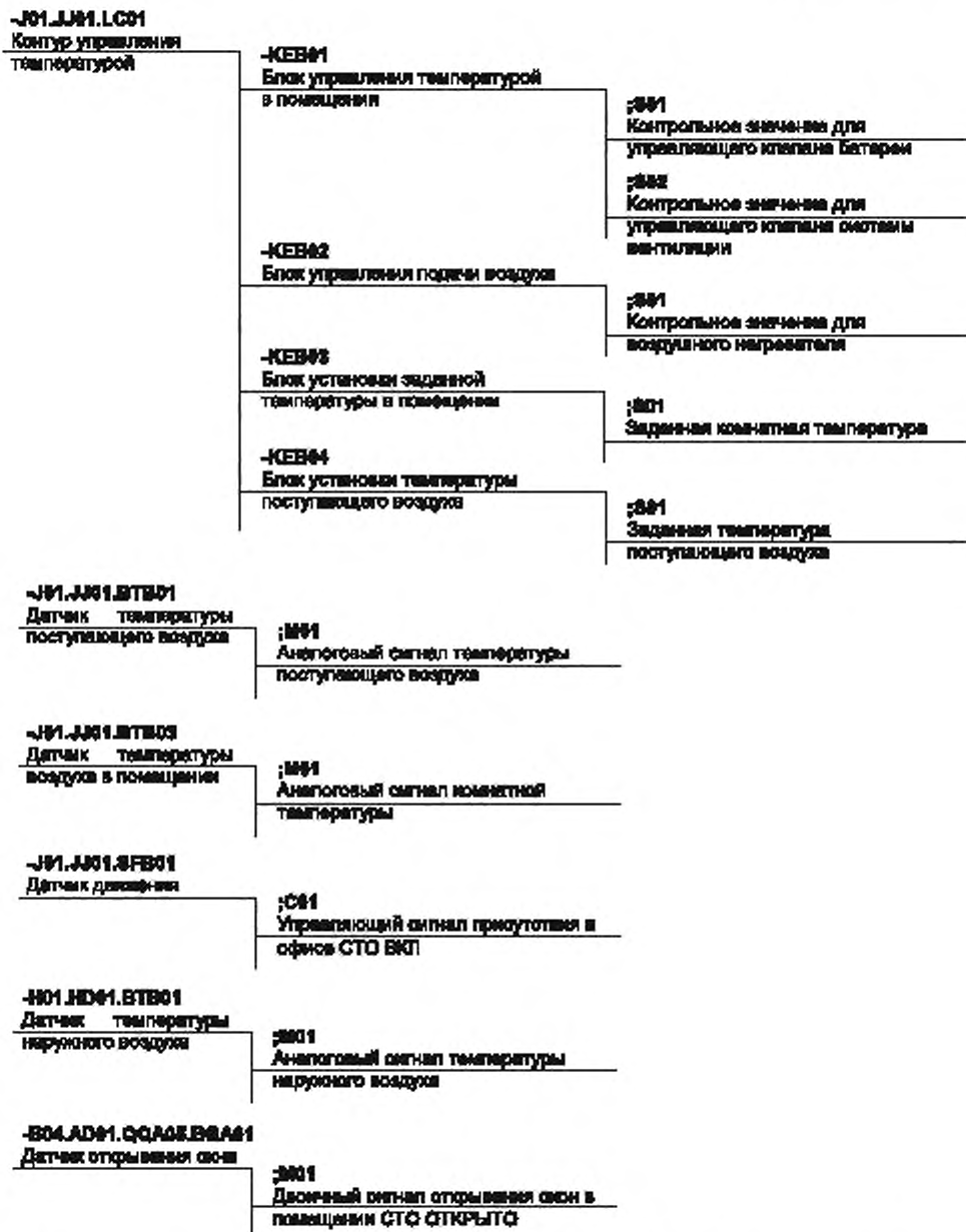
Рисунок В.15 — Древоидная функционально-ориентированная структура представления системы управления инженерными системами помещения (с обозначением системных сигналов)
