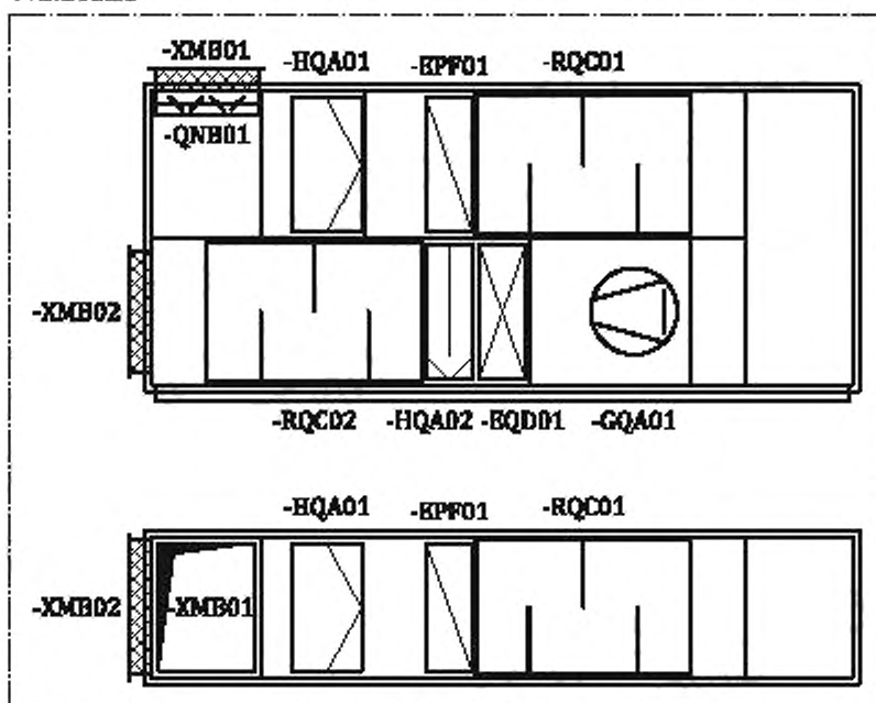
Рисунок В.12 — Схема вентиляционной установки
