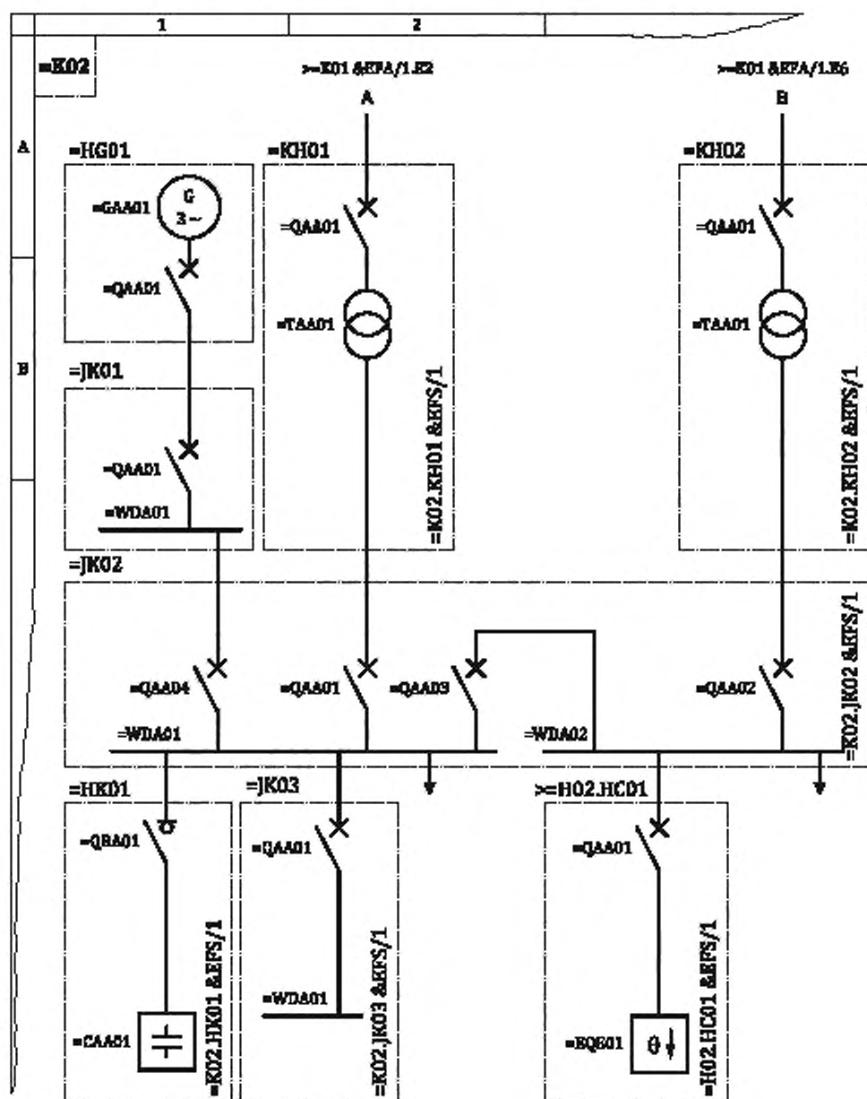
Рисунок В.19 — Схема распределения слаботочной системы
