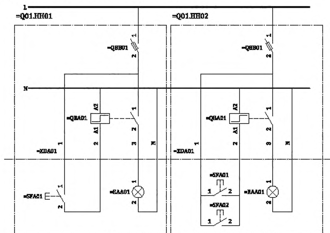
Рисунок В.21 — Схематичное отображение объектов системы освещения
