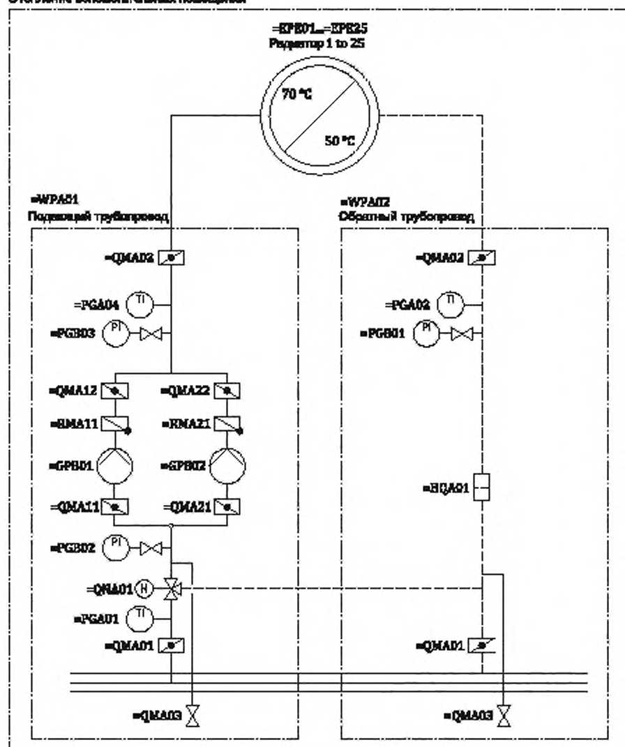
Рисунок В.17 — Принципиальная схема системы отопления
