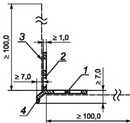
Рисунок 2 — Профиль-капельник с щелочестойкой стеклосеткой
