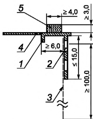
Рисунок 3 — Примыкающий оконный профильный элемент с щелочестойкой стеклосеткой
