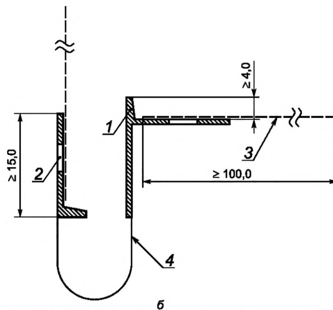
Рисунок 6 — Е-образный (а) и V-образный (б) деформационные профильные элементы
