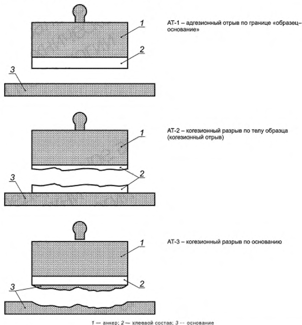
Рисунок 1 — Основные характерные виды отрыва образцов при определении прочности сцепления с основанием
