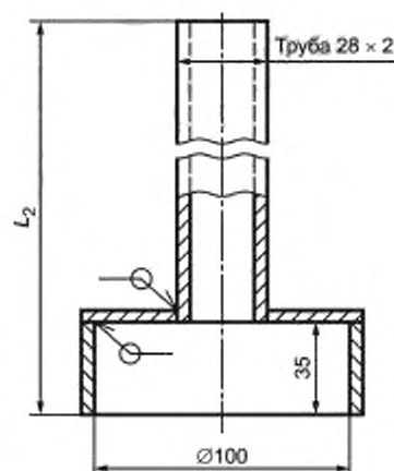
Рисунок Г.2 — Направляющая
