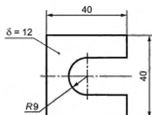
Рисунок Г.3 — Платик
