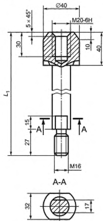
Рисунок Г.1 — Фиксатор для съемных деталей
