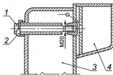
1 — болт; 2 — отгибная шайба; 3 — борт; 4 — вкладыш
