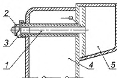
1 — шпилька; 2 — гайка; 3 — отгибная шайба; 4 — борт; 5 — вкладыш
