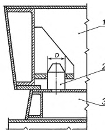
1 — щит; 2 — штырь; 3 — рамка
