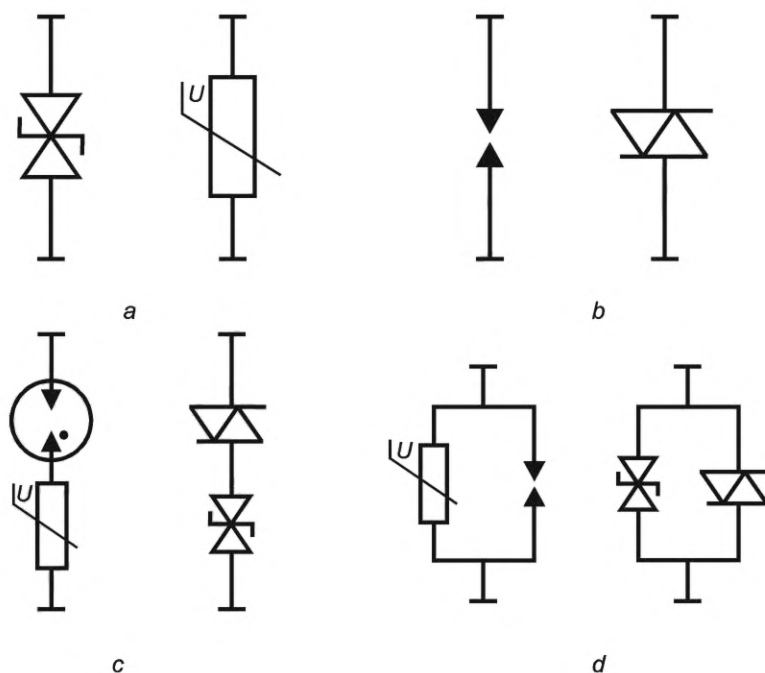
a — компоненты, ограничивающие напряжение; b — компоненты, коммутирующие напряжение; c — компоненты, ограничивающие напряжение, включенные последовательно с коммутирующими напряжением компонентами; d — компоненты, ограничивающие напряжение, включенные параллельно с коммутирующими напряжением компонентами
