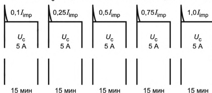
Рисунок А.3 — Схема временных характеристик испытания для дополнительных пяти импульсов
