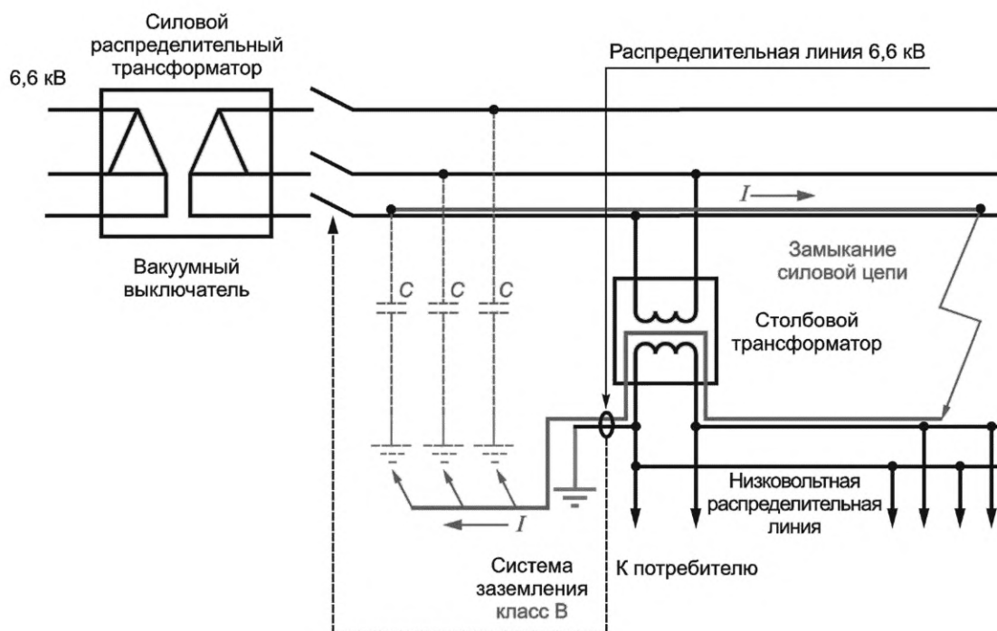
Рисунок Е.12 — Типовая конфигурация энергосистемы Японии
