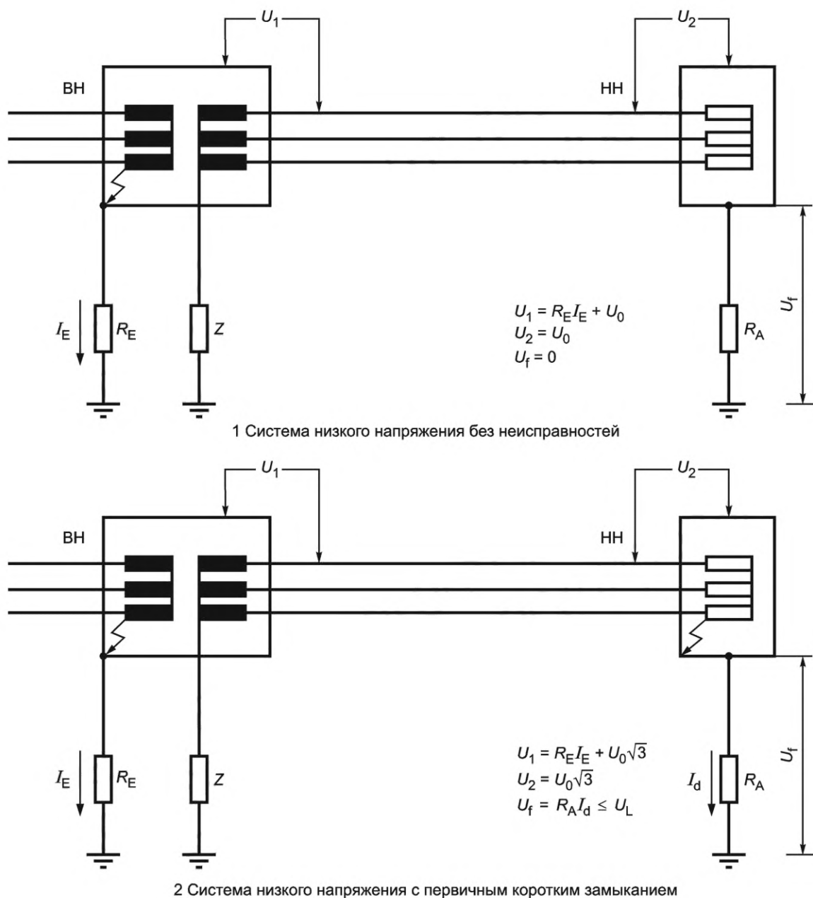
Рисунок Е.7 — Система IT, пример с1 (IEC 60364-4-44:2007, рисунок 44Е)
