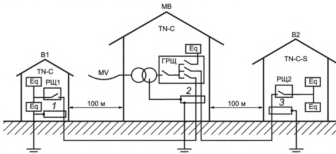
B1, B2 — здание 1, 2; MB — главное здание; 1, 2, 3 — шина заземления; ГРЩ — главный распределительный щит; РЩ — распределительный щит; Eq — оборудование нагрузки
