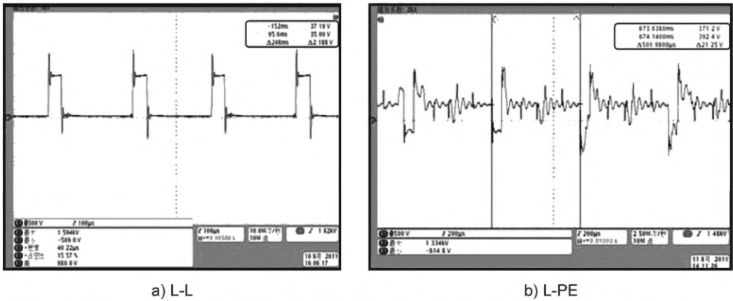
Рисунок G.6 — Напряжение ШИМ между генератором и преобразователем в цепи ротора
