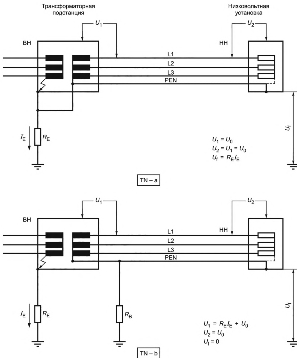
Рисунок Е.3 — Система TN (IEC 60364-4-44:2007, рисунок 44В)
