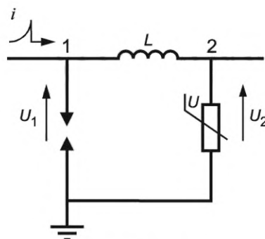
Рисунок F.3 — Пример координации УЗИП на основе разрядника и УЗИП на основе металлооксидных варисторов (МОВ)
