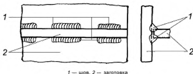
Рисунок 2 — Цепной прерывистый шов
