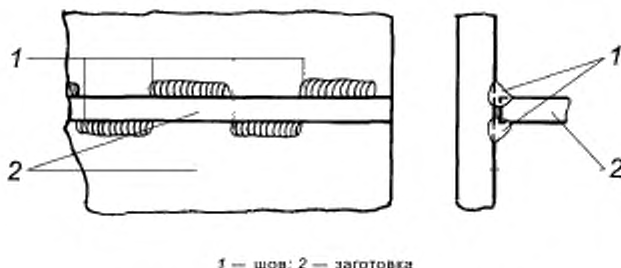
Рисунок 1 — Шахматный прерывистый шов
