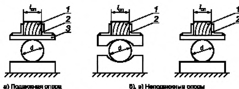
1 — деревянный брусок; 2 — стальной уголок; 3 — стальная пластина
