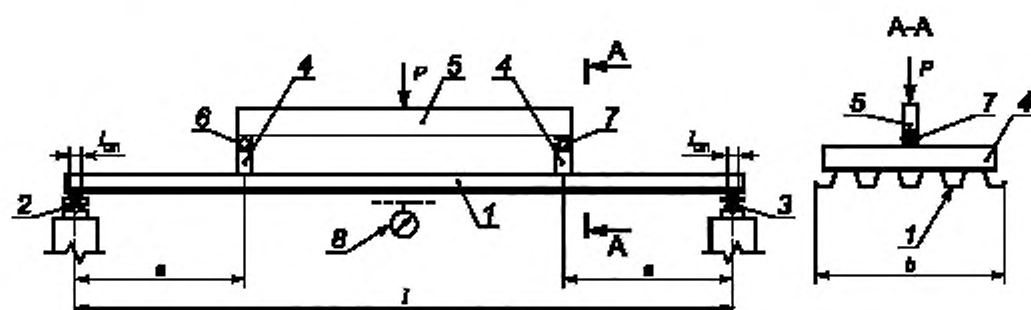
1 — испытываемый образец; 2 — неподвижная опора стэнда; 3 — подвижная опора стэнда; 4 — поперечная распределительная балка; 5 — траверса; 6 — неподвижная опора траверсы; 7 — подвижная опора траверсы; 8 — индикатор прогиба
