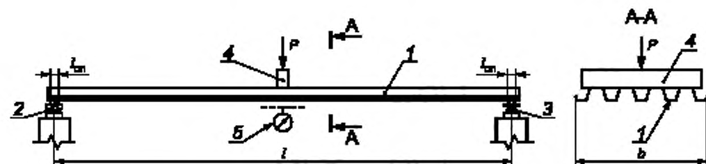
1 — испытываемый образец; 2 — неподвижная опора стэнда; 3 — подвижная опора стэнда; 4 — поперечная распределительная балка; 5 — индикатор прогиба
