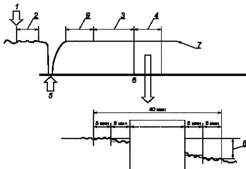
Рисунок D.2 — Стационарное испытание теплопроизводительности с размораживанием в конце периода предварительной подготовки
