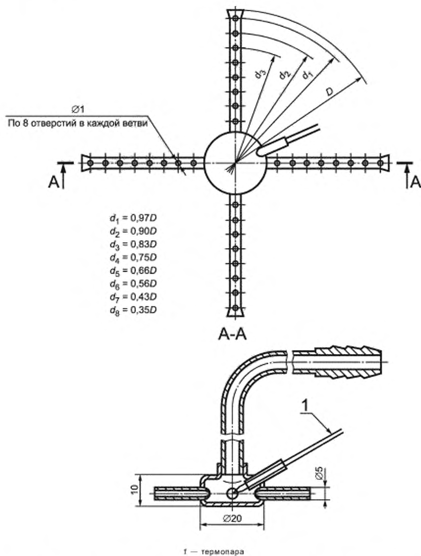
Рисунок 8 — Устройство для отбора проб и измерения температуры продуктов сгорания для дымоходов диаметром D \geq 100 мм (приборы типа В).
