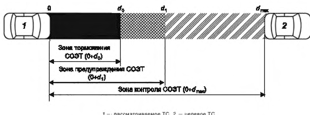
Рисунок 3 — Зоны системы опережающего экстренного торможения
