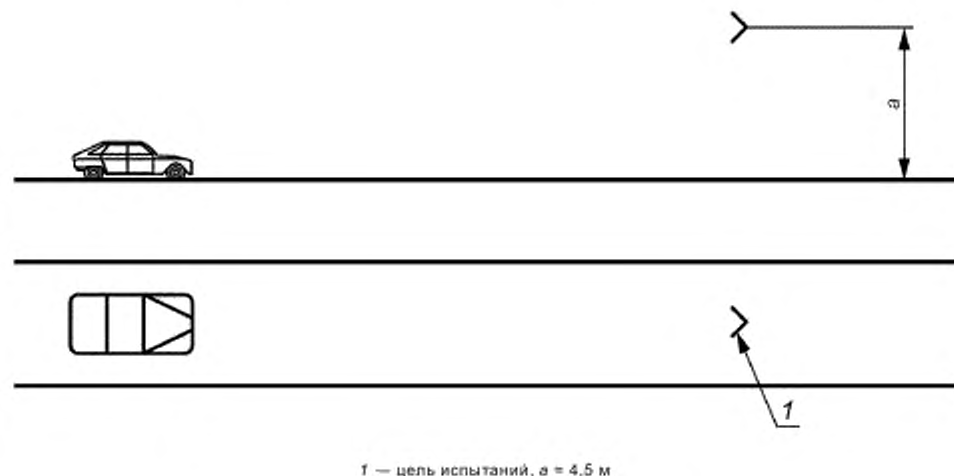
Рисунок А.1 — Испытание на ложное реагирование (объект сверху)
