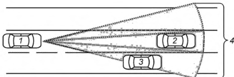
1 — РТС; 2 — ЦТС на полосе движения РТС; 3 — ТС на соседней с РТС полосе движения; 4 — зона контроля (серый фон); — — — — — основная зона предупреждения, * * * — дополнительная (правая боковая) зона предупреждения при включенном на РТС указателе правого поворота; . . . — дополнительная (левая боковая) зона предупреждения при включенном на РТС указателе левого поворота
