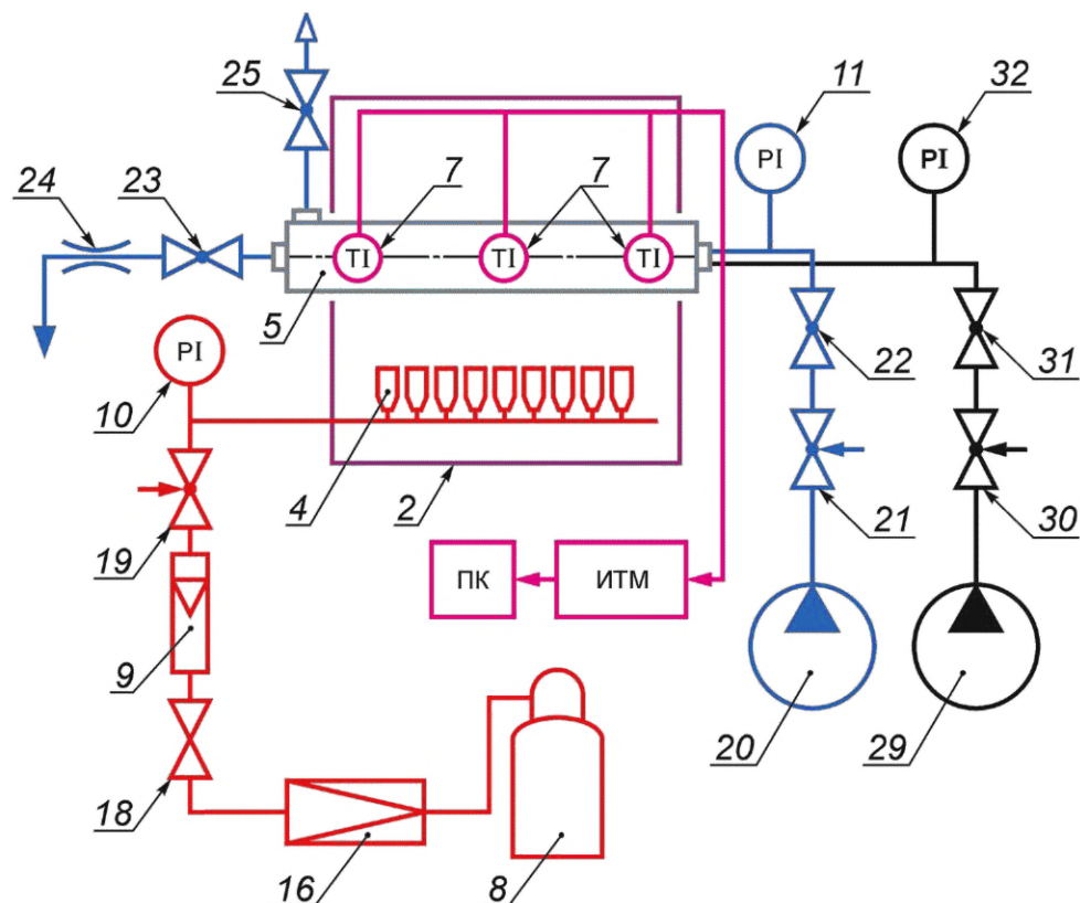
2 — испытательная камера; 4 — газовые горелки; 5 — трубопроводная сборка; 7 — термодатчики (ТИ); 8 — газовый баллон; 9 — расходомер; 10, 11, 32 — манометры (PI); 16 — редуктор; 18, 22, 23, 25, 31 — краны; 19, 21, 30 — регулирующие устройства; 20 — источник гидравлического давления; 24 — диафрагма; 29 — источник пневматического давления; ПК — персональный компьютер; ИТМ — многоканальный технологический измеритель
