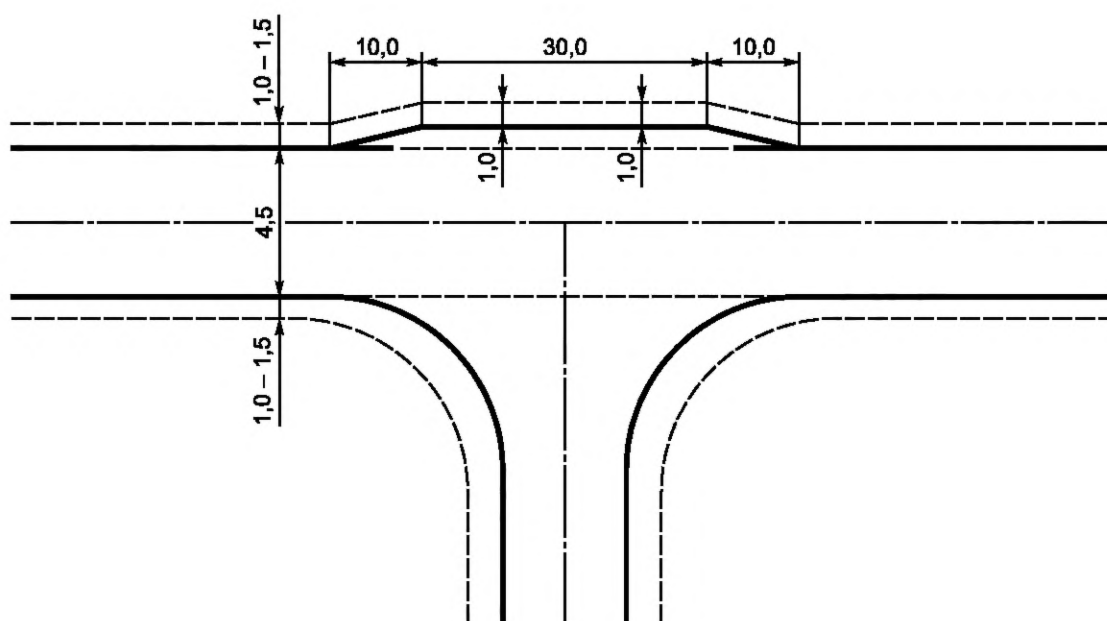
в) Карман в зоне примыкания
