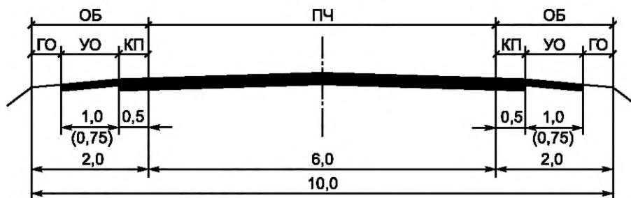
а) Типовой поперечный профиль автомобильной дороги категории IV A-р, IVA-п и IVБ-п
