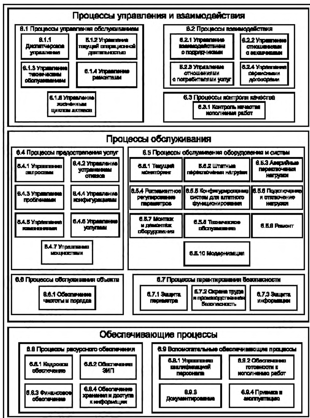
Рисунок 1 — Процессы операционной модели эксплуатации инженерной инфраструктуры ЦОД
