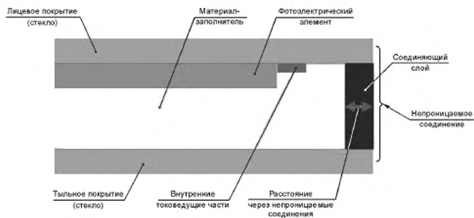
Рисунок А.3 — Пример фотоэлектрического модуля типа «стекло/стекло» с непроницаемыми соединениями
