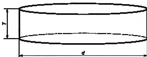
d — максимальный диаметр плавучей платформы или КСС; T — осадка полностью нагруженного КСС
