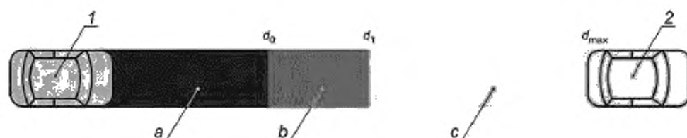
1 — ТС; 2 — ЦТС; а — обнаружение не требуется; б — требуется обнаружение ЦТС; с — требуется определение расстояния
