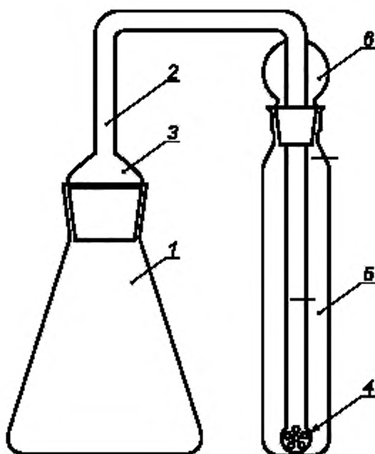
1 — реакционный сосуд, представляющий собой коническую колбу вместимостью 100 или 150 см 3 со шлифом и меткой, соответствующей объему 50 см 3 ; 2 — отводная трубка с хвостом 29 мм; 3 — расширение для ваты, пропитанной раствором уксуснокислого свинца; 4 — барботер, предназначенный для лучшего поглощения арсина; 5 — пробирка вместимостью 20 или 25 см 3 и высотой не менее 15 см для поглотительного раствора; 6 — отверстие диаметром не более 2 мм в расширенной части отводной трубки, соединенной с пробиркой, для исключения разгерметизации установки во время отгонки арсина
