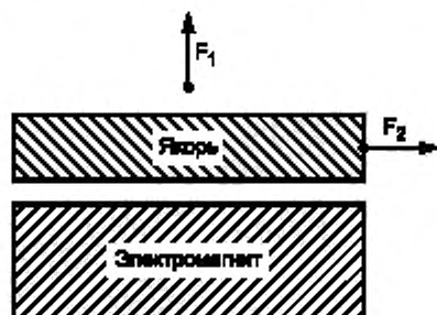
F_1 — сила отрыва в удерживающих замках F_2 — сила сдвига в сдвиговых замках
