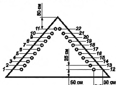
Рисунок 2 — Схема отбора проб из конической насыпи
