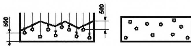
Рисунок 4 — Схема отбора проб от неконусообразной насыпи
