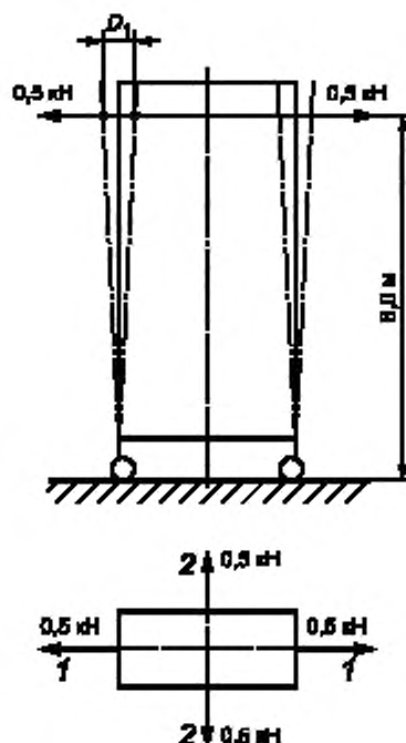
1 — первое испытание в двух противоположных направлениях; 2 — второе испытание в двух противоположных направлениях
