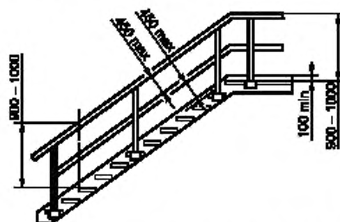
Рисунок 4 — Геометрические параметры защитного ограждения маршевой лестницы
