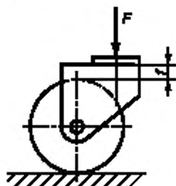
Рисунок 7 — Схема испытания колеса подмости на прочность
