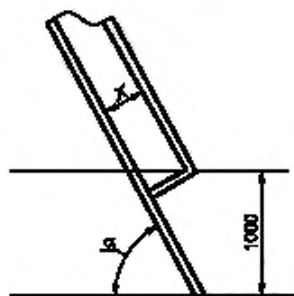
Рисунок 4 — Геометрические параметры защитного ограждения маршевой лестницы
