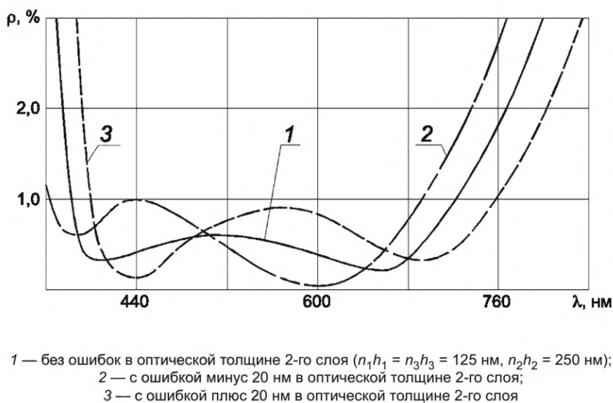
Рисунок К.2 — Кривые спектральных коэффициентов отражения \rho(\lambda) трехслойных покрытий с ошибками и без ошибок в оптической толщине 2-го слоя
