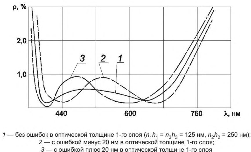
Рисунок К.1 — Кривые спектральных коэффициентов отражения \rho(\lambda) трехслойных покрытий с ошибками и без ошибок в оптической толщине 1-го слоя
