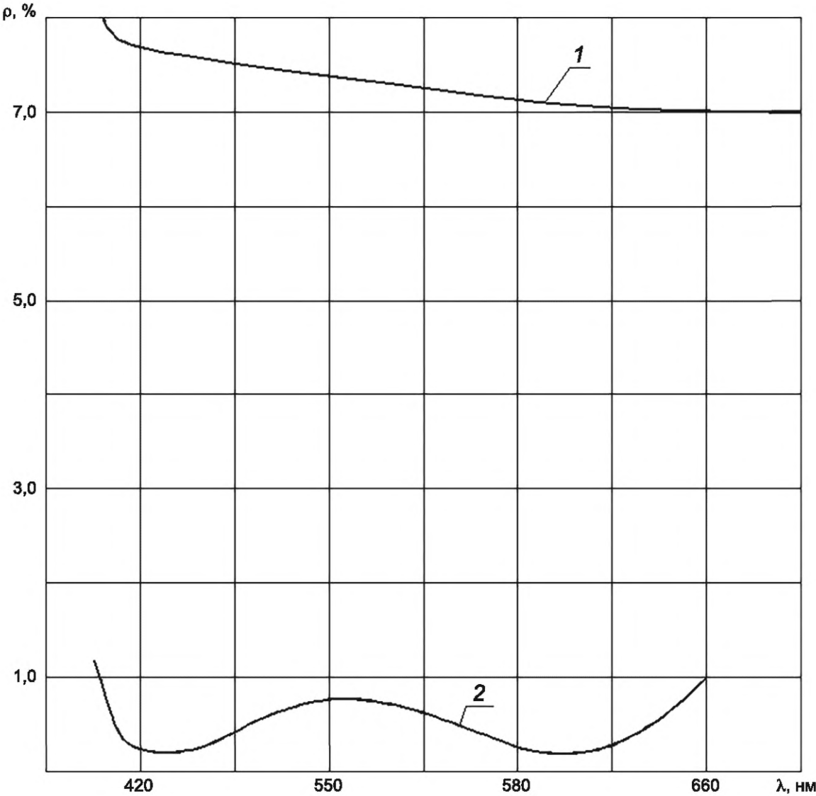
1 — детали из стекол марки ТФ7 с покрытием 200.45P.46P.43P.280; 2 — детали из стекол марки ТФ7 без покрытия
