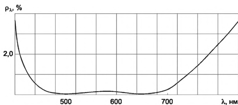
а) Спектральный диапазон просветления от 430 до 750 нм
