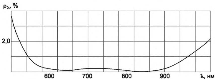
б) Спектральный диапазон просветления от 580 до 920 нм
