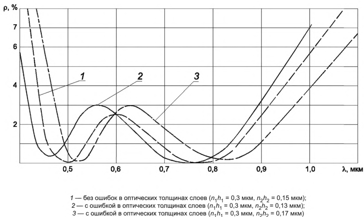
Рисунок Ж.1 — Кривые спектральных коэффициентов отражения \rho(\lambda) от поверхности стекла марки К8 с двухслойным ахроматическим покрытием 44Р.43Р
