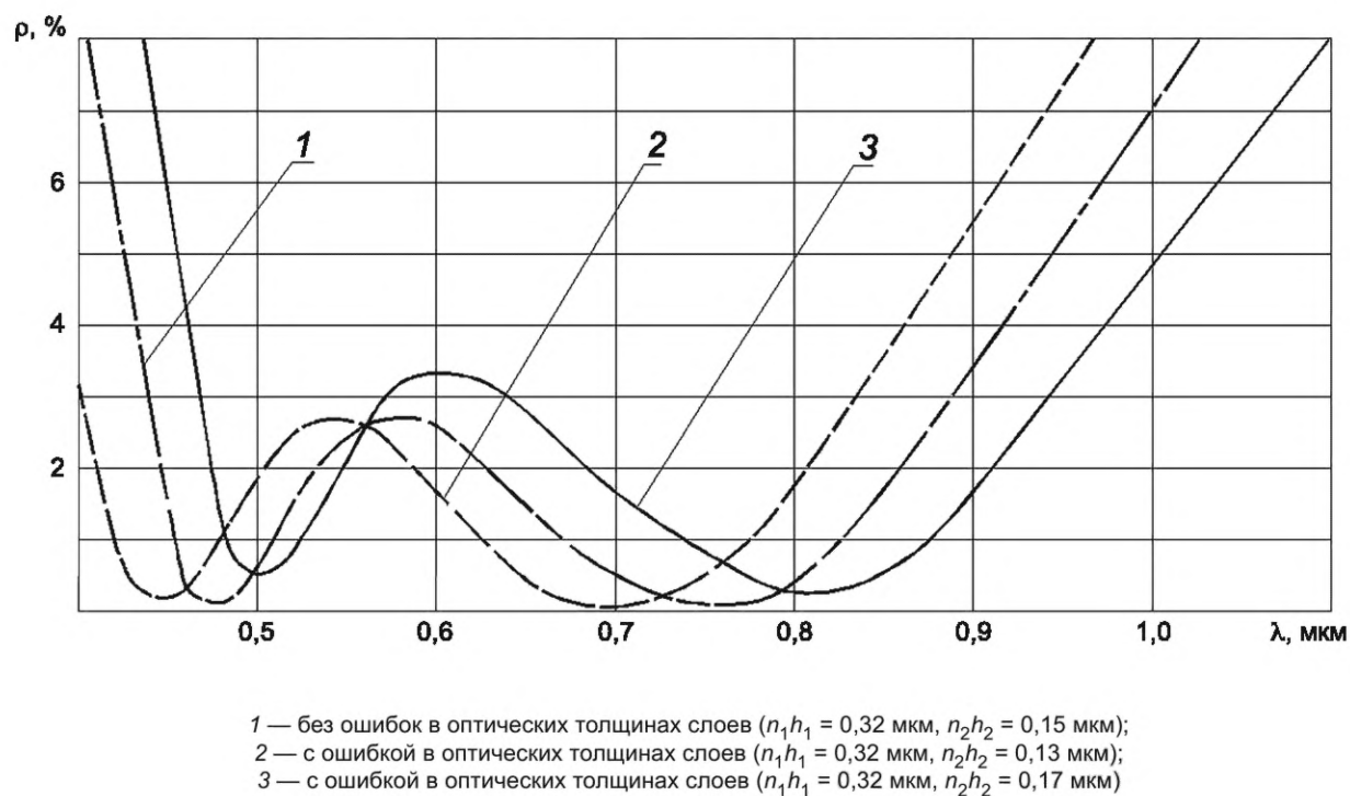
Рисунок Ж.2 — Кривые спектральных коэффициентов отражения \rho(\lambda) от поверхности стекла марки К8 с двухслойным ахроматическим покрытием 44P.43P
