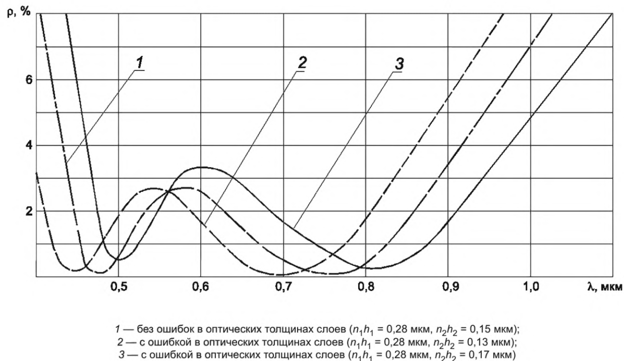
Рисунок Ж.3 — Кривые спектральных коэффициентов отражения \rho(\lambda) от поверхности стекла марки К8 с двухслойным ахроматическим покрытием 44P.43P
