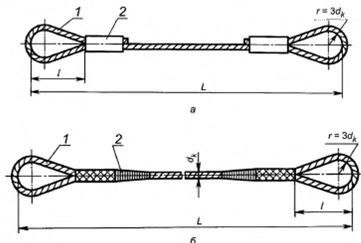
Рисунок 6 — Петлевой канатный строп исполнения 1 с заделкой концов каната опрессовкой алюминиевой втулкой (а) и с заделкой концов каната заплеткой (б)
