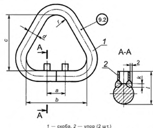
Рисунок Б.22 — Звено Т грузоподъемностью свыше 12,5 тс
