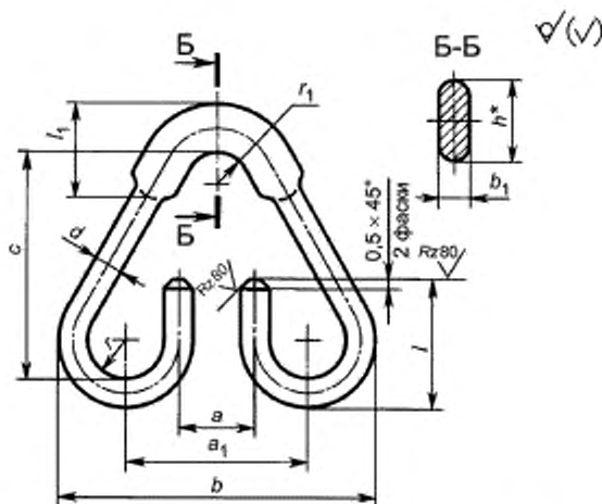
Рисунок Б.10 — Скоба Ст4 для звеньев Рт4
