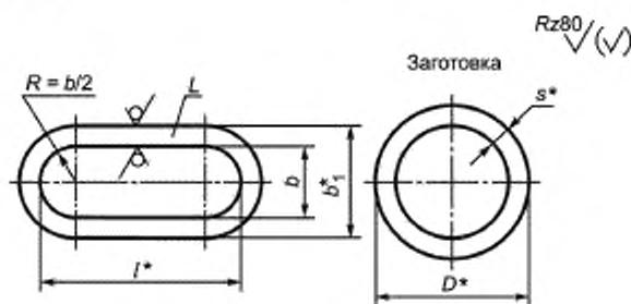
Рисунок В.3 — Стальная втулка СВт
