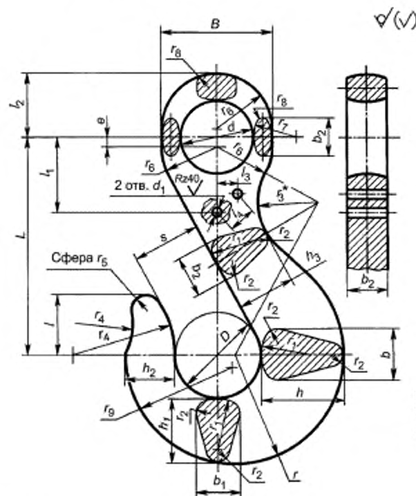
Рисунок Б.35 — Чалочный крюк Кч2 для захвата К2
