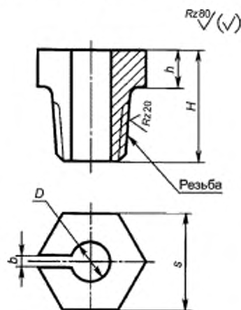
Рисунок Б.12 — Гайка Г для звеньев Рт4
