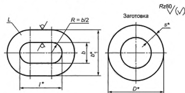
Рисунок В.2 — Аллюминиевая втулка Вт
