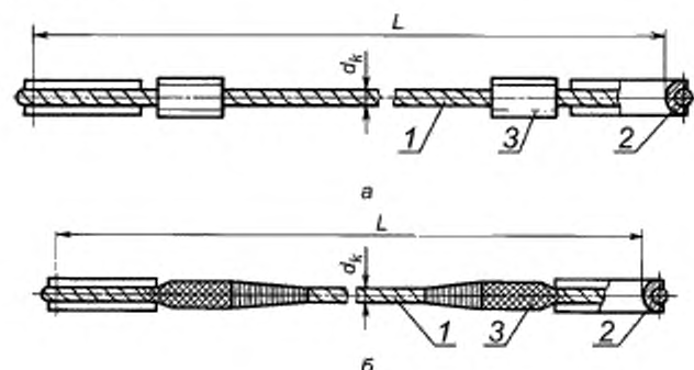
Рисунок А.1 — Канатная ветвь с заделкой концов каната опрессовкой алюминиевой или стальной втулкой (а) и с заделкой концов каната заплеткой (б)
