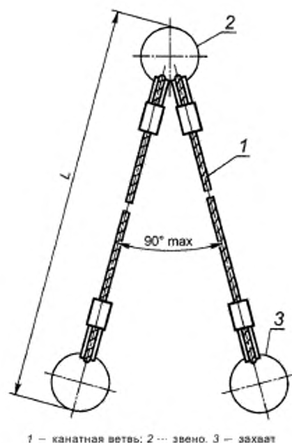
Рисунок 2 — Двухветвевой канатный строп
