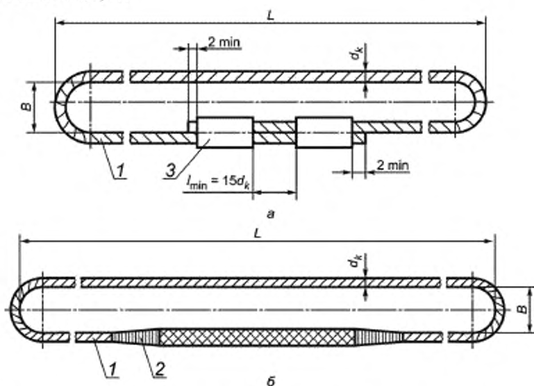
1 — стальной канат грузового назначения марки 1, нераскручивающийся; 2 — место заделки концов каната; 3 — втулка (2 шт.); d_k — диаметр каната
