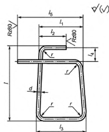
Рисунок Б.36 — Замок 32 для захвата К2
