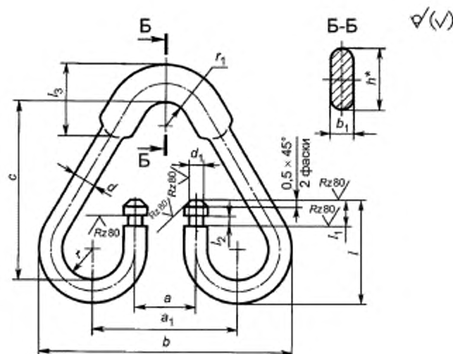
Рисунок Б.8 — Скоба СтЗ для звеньев РтЗ
