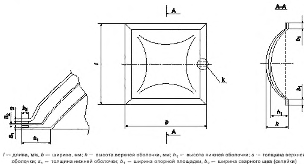
Рисунок А.3 — КПМ для установки с помощью рамы (тип Р)
