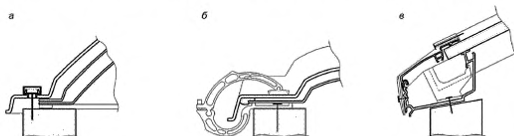
Рисунок Б.1 — Крепление КПМ к основанию фонаря шайбами с защитными колпачками — Ш (а), винтовыми прижимами — В (б), прижимной рамой (в)
