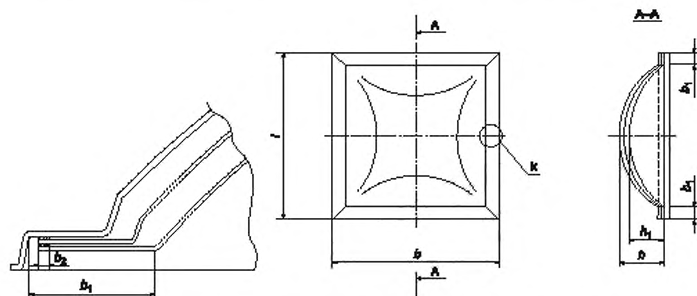
Рисунок А.1 — КПМ с отверстиями по контуру для установки с помощью защитных колпачков (тип Ш)
