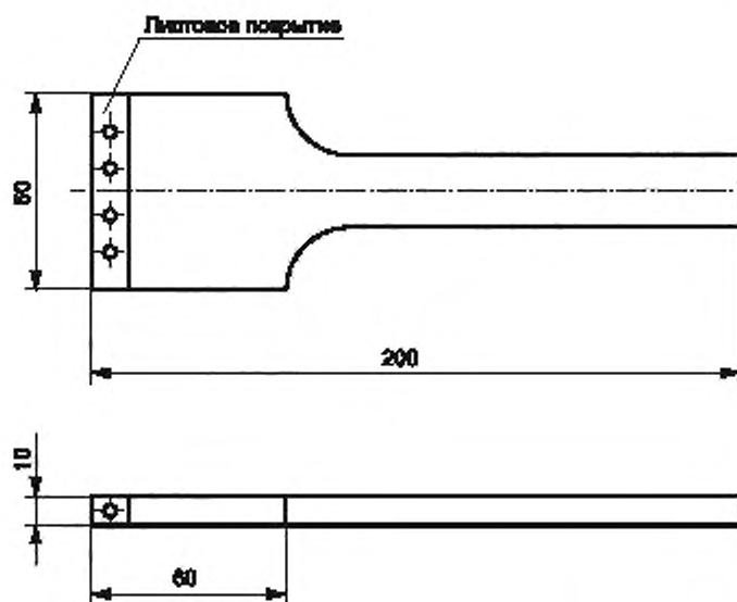
Рисунок 4 — Шпатель для уплотнения растворной смеси
