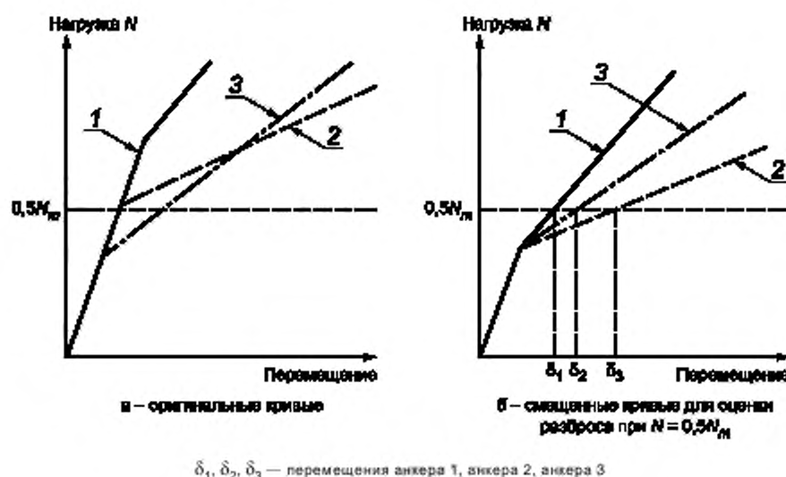
Рисунок 12 — Исходные и трансформированные диаграммы испытания анкеров
