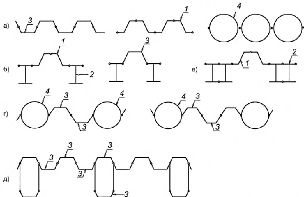
а) Стена, состоящая из корытных шпунтовых свай (типа Ларсен и др.), Z-образного шпунта, трубойшпунта; б) Стена, состоящая из модулей, включающих одну двутавровую и две Z-образные или одну корытную шпунтовую сваи; в) Стена, состоящая из модулей, включающих две двутавровые и две Z-образные или одну корытную шпунтовую сваи; г) Стена, состоящая из модулей, включающих трубойшпунт и две или три корытные шпунтовые сваи; д) Стена, состоящая из модулей, включающих коробчатый элемент и пять корытных шпунтовых свай.
