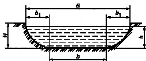
Рисунок 5 — Комбинированная форма поперечного сечения каналов проводящей сети
