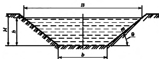
B — ширина поверху, м; b — ширина канала по дну, м; h — глубина воды в канале, м; H — глубина канала, м; m — коэффициент заложения откоса ( m = \text{ctg} \theta , \theta — угол наклона откоса)
