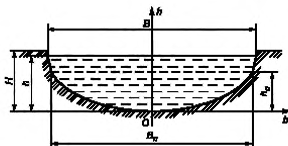
Рисунок 4 — Полигональная форма поперечного сечения каналов проводящей сети
