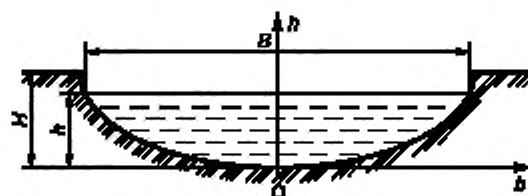
B — ширина поверху, м; H — глубина канала, м; h — глубина воды в канале, м
