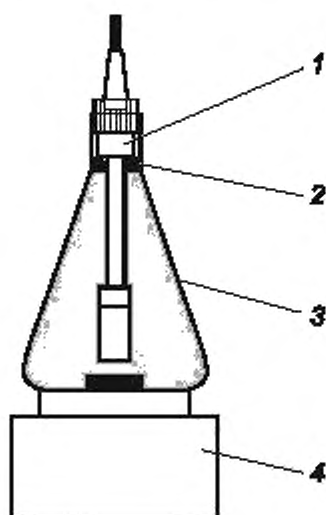
1 — датчик; 2 — резиновое кольцо; 3 — склянка; 4 — магнитная мешалка
