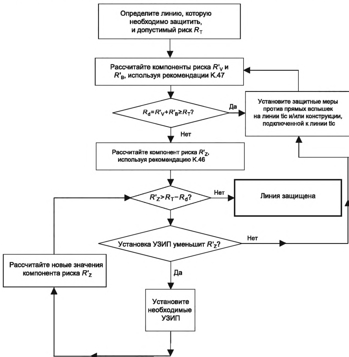
Рисунок С.1 — Процедура оценки рисков
