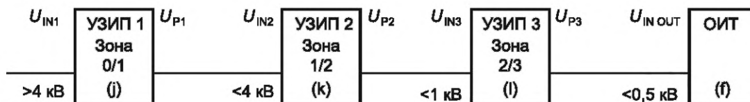
Рисунок 5 — Пример конфигурации по зонам (см. рисунок 4)
