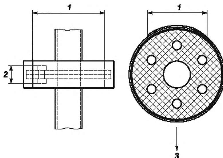
Рисунок В.1 — Пример установки брызгозащитного кожуха фланца
