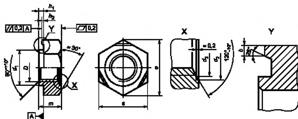
Рисунок 1 — Размеры гаек
