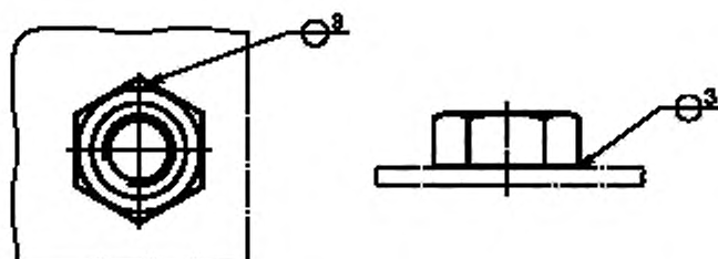
Рисунок 2 — Указание мест сварки в чертежах
