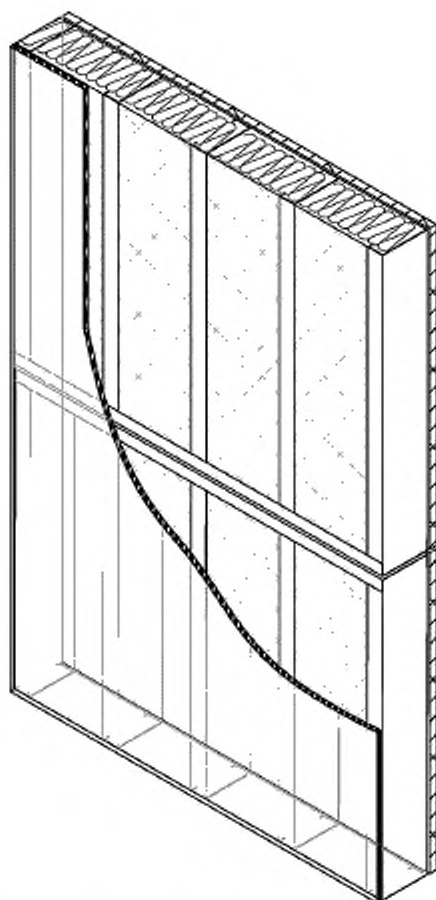
Рисунок 11 — Фрагмент КОС из модуля полной заводской готовности (МЗГ)
