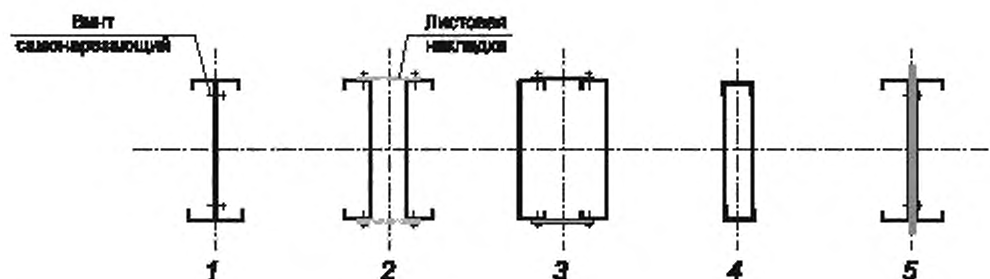
Рисунок А.1 — Одиночные сечения стоек каркаса КОС
