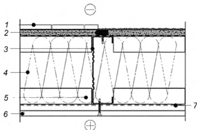
1 — облицовка (фасадная отделка); 2 — самонарезающие винты для соединения обшивок с элементами каркаса; 3 — стойки каркаса стены; 4 — основной теплоизоляционный слой (между стойками каркаса); 5 — противоусадочные уголки; 6 — внутренняя обшивка КОС; 7 — пароизоляция
