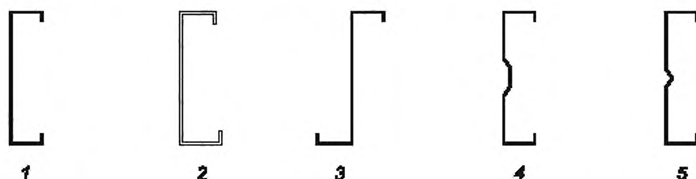
Рисунок А.1 — Одиночные сечения стоек каркаса КОС
