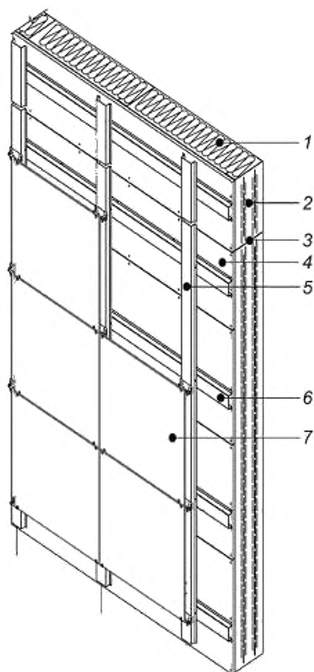
1 — основной теплоизоляционный слой (между стойками каркаса); 2 — стойки каркаса стены; 3 — стык модульной конструкции КОС; 4 — наружная обшивка КОС; 5 — стальные профили обрешетки (вертикальные), 6 — стальные профили обрешетки (горизонтальные); 7 — облицовка (фасадная отделка)
