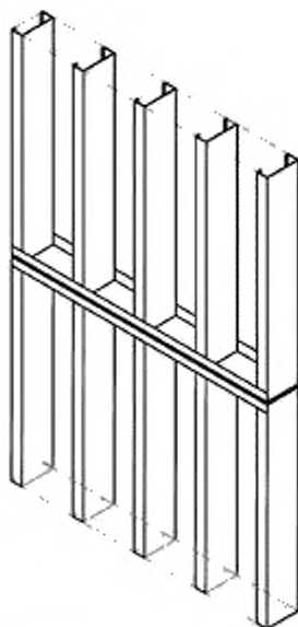
Рисунок 13 — Фрагмент КОС из каркасного модуля (МНК)
