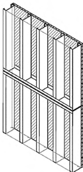
Рисунок 12 — Фрагмент КОС из модуля с наружной обшивкой (МНО)
