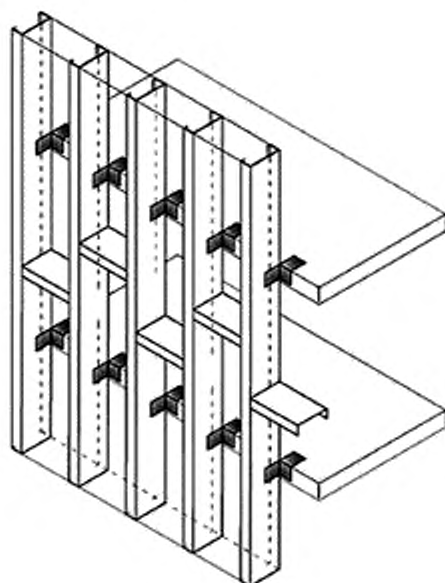
а) Стоечно-ригельный способ
