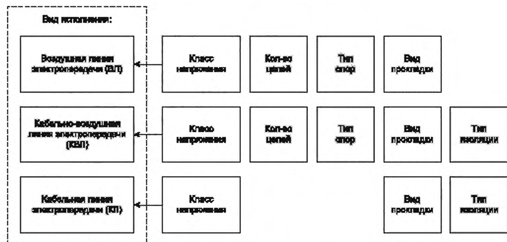
Рисунок А.3 — Структура набора атрибутов единицы оборудования «Линия электропередачи»
