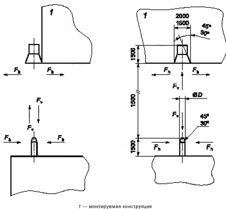
Рисунок А.2 — Направляющий штырь и ловитель
