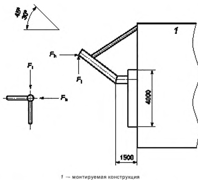
Рисунок А.3 — Горизонтальный рогаобразный скользящий кранец с вертикальным направляющим устройством
