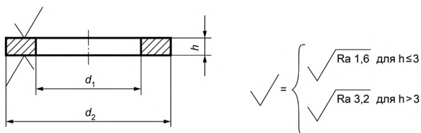
Рисунок 1 — Размеры
