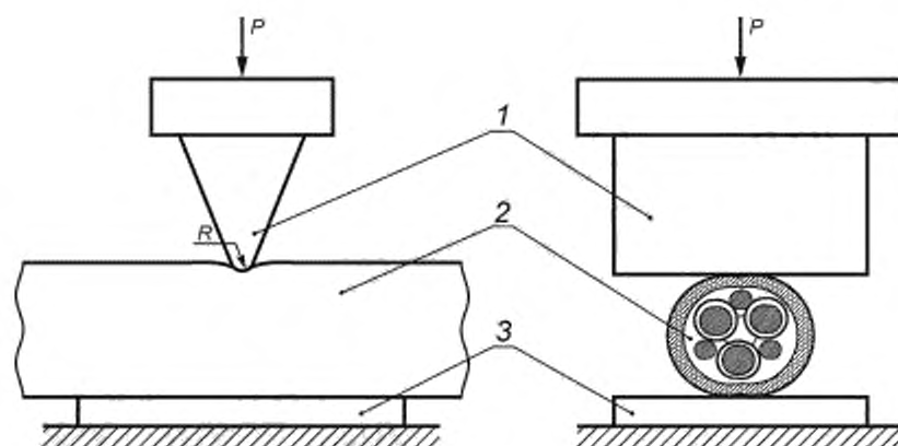
Рисунок 1 — Схема стенда на раздавливание гибкого шахтного кабеля
