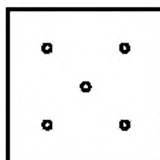
Рисунок 3 — Схема расположения точек измерения твердости материала рукава
