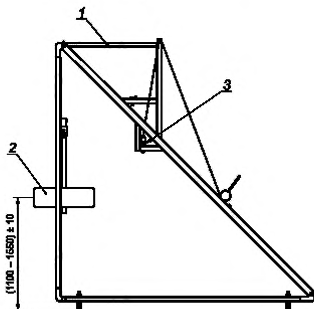
1 — рама стенда, 2 — колесо с грузом, 3 — спусковой замок
