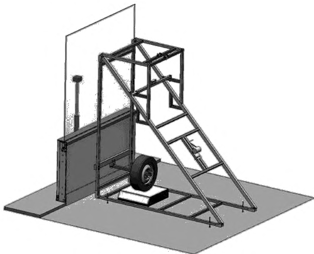
Рисунок 3 — Исходное положение маятника для проведения взвешивания
