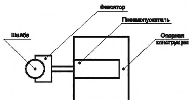
Рисунок 2 — Схематическое изображение установки «шайбомет»
