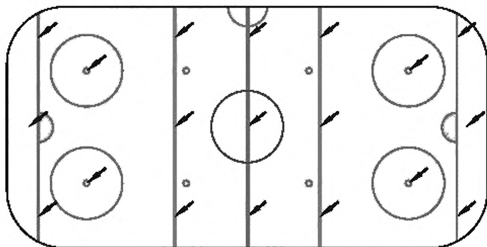
Рисунок Б.1 — Схема расположения точек контрольных замеров температуры поверхности искусственного льда
