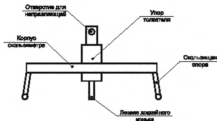
Рисунок 4 — Схематическое изображение скользящего устройства
