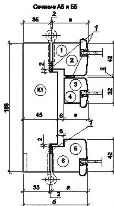
1 — уплотнительный профиль
