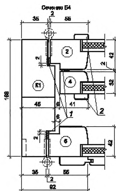
1 — уплотнительный профиль, 2 — наличник
