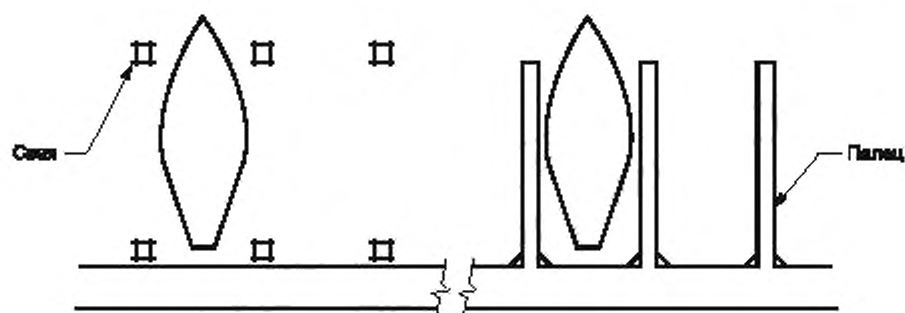
Рисунок 3 — Причальное сооружение для одного судна
