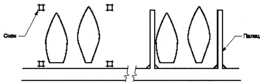
Рисунок 4 — Причальное сооружение на два судна
