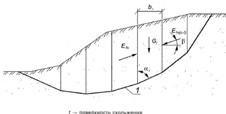
Рисунок Б.1 — Схема к расчету общей устойчивости при поступательном перемещении
