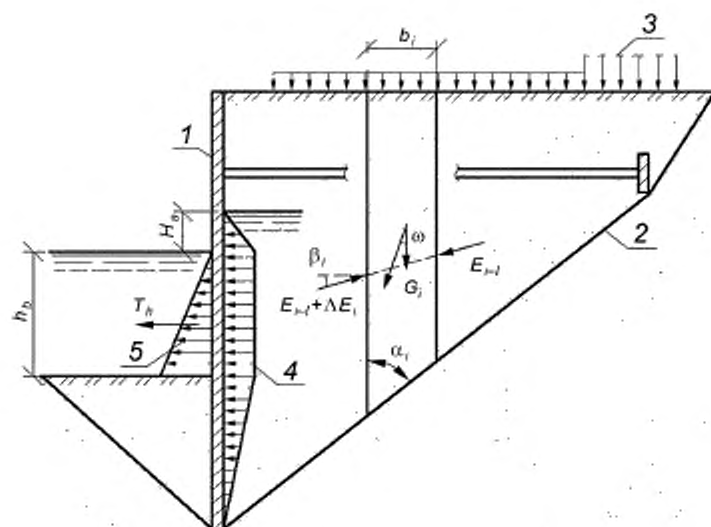
1 — набережная, 2 — возможная поверхность сдвига, 3 — нагрузка на поверхности грунта, 4 — давление фильтрующей воды, 5 — сейсмическое давление воды акватории
