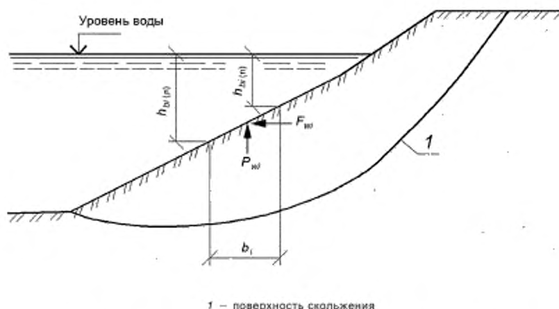
Рисунок Е.2 — Схема к расчету сейсмического давления свободной воды
