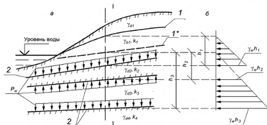
а — Расчетная схема; б — Эпюра давления воды в сечении I—I 1, 1* и 2 — то же, что и на рисунках Ж.1 и Ж.2; k_1 > k_2, k_3 > k_4
