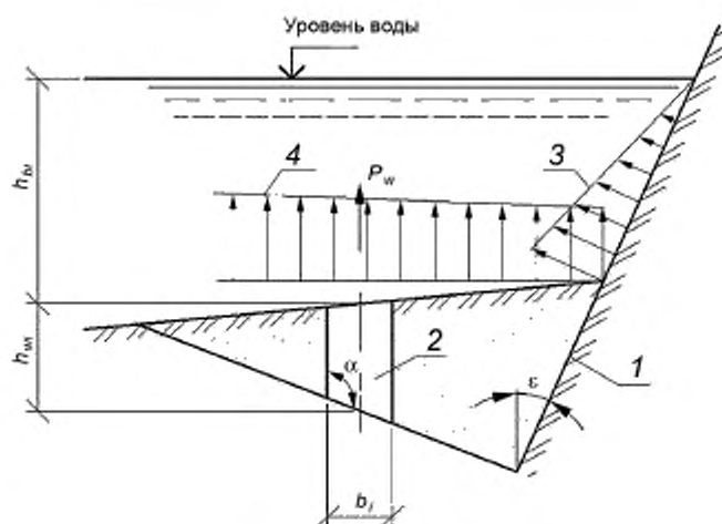
1 — расчетная поверхность; 2 — вертикальный элемент призмы выпора; 3 — эпюра сейсмического давления воды на поверхность стены, контактирующей с водой; 4 — эпюра сейсмического давления воды на поверхность грунта
