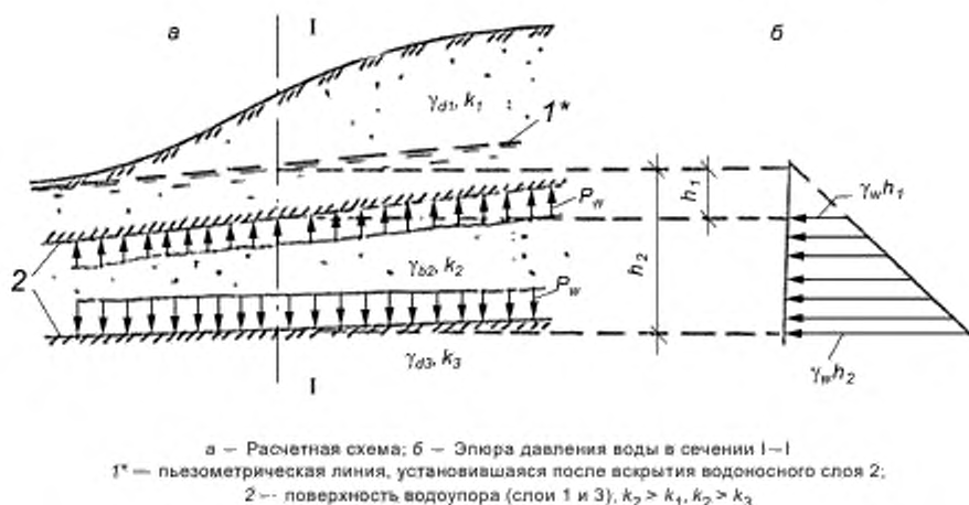
Рисунок Ж.2 — Схема к определению нагрузок от фильтрующей воды при напорной фильтрации
