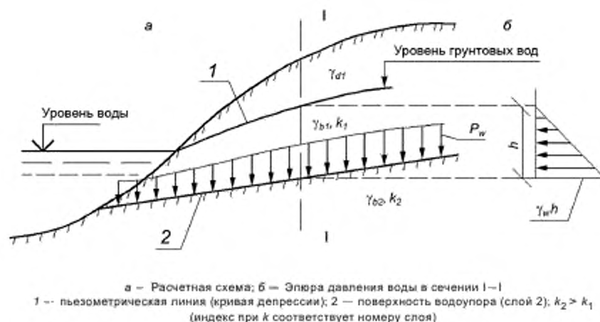
Рисунок Ж.1 — Схема к определению нагрузок от фильтрующей воды при безнапорной фильтрации
