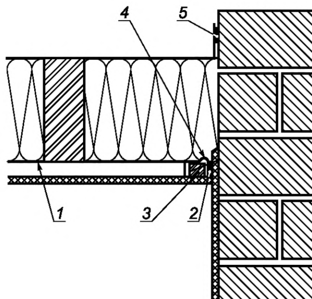
1 — пароизоляционная пленка; 2 — двусторонняя соединительная лента; 3 — прижимной брус; 4 — компенсационная складка из пароизоляционной пленки; 5 — клей для водозащитной пленки
