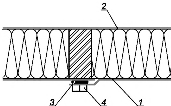
1 — пароизоляционная пленка; 2 — диффузионная пленка; 3 — соединительная лента; 4 — прижимной брус
