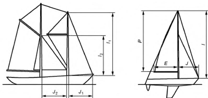
l — высота переднего треугольного паруса, J — база переднего треугольного паруса; P — высота главного паруса; E — база главного паруса
