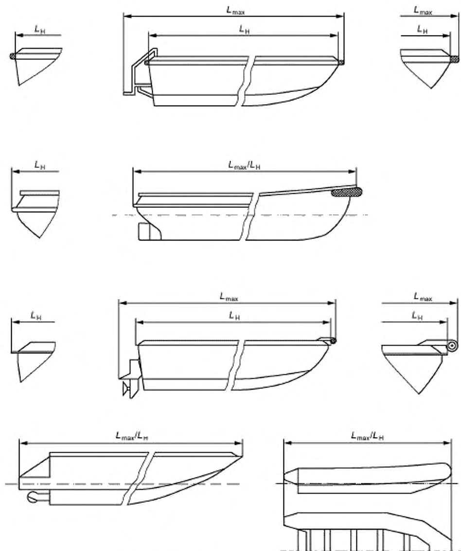
а) Определение L_{max} и L_H для непарусных судов
