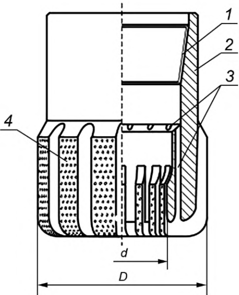
1 — присоединительная резьба; 2 — корпус; 3 — промывочные каналы; 4 — лопасти с покрытием из природных или синтетических алмазов или СКМ; D — внешний номинальный диаметр бурильной головки; d — диаметр керна
