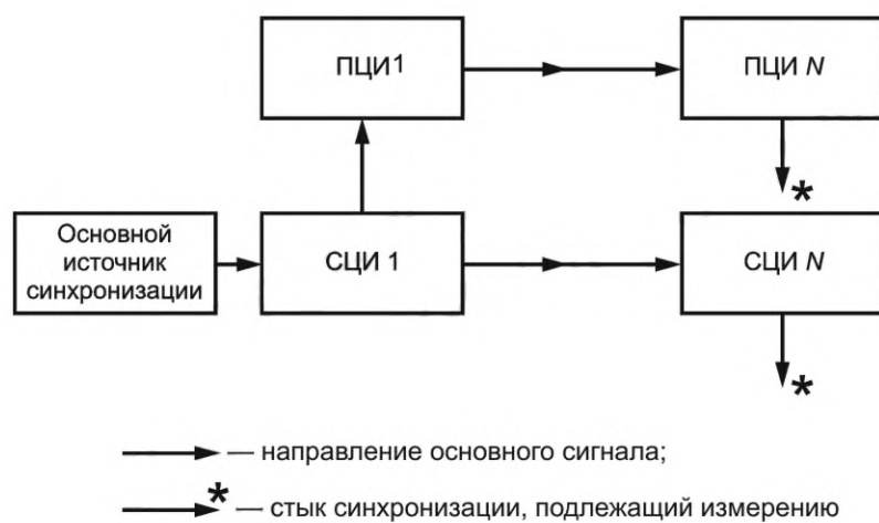
Рисунок Б.2 — Стык Т4 или Е1 на выходе аппаратуры СП СЦИ/ПЦИ (основной источник синхронизации)
