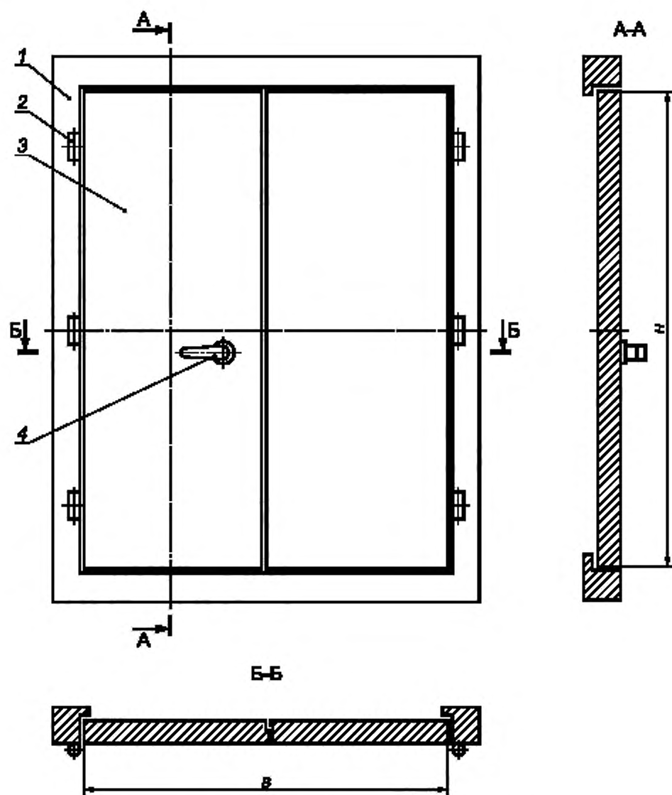
Рисунок А.4 — Двустворчатая дверь глухая симметричная
